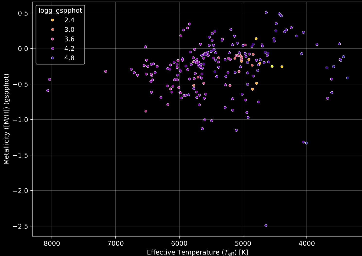
APOGEE DR17 Field: [200-60] Stellar Population Parameters (n= 211)
